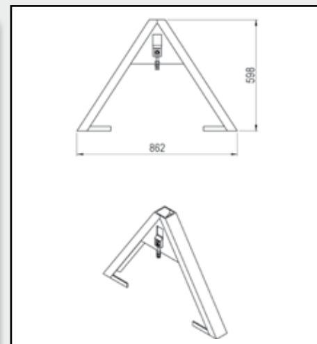
Triangle d'attelage: CAT 1
