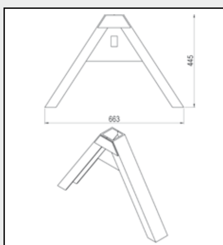
Triangle d'attelage: CAT 0
