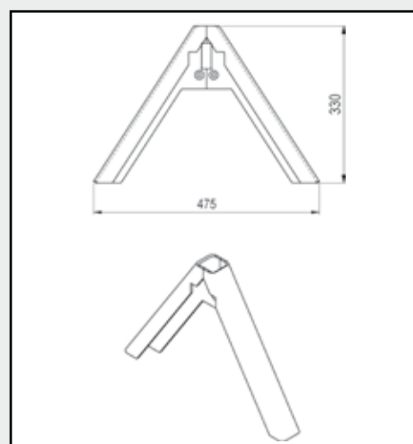
Triangle d'attelage: CAT communal
